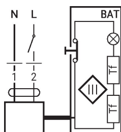
AC 230 V, Zamknij/Otwórz
