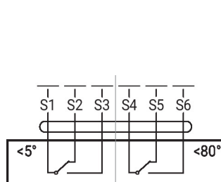
Styk pomocniczy
