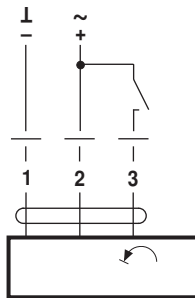
DR(C)24G(..)-5 DR(C)24G(..)-7
