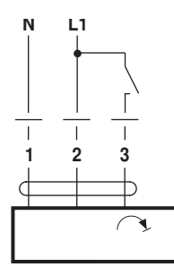
GR(C)230G(..)-5 GR230G(..)-7
