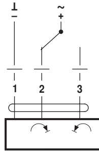
GR24G(..)-7
