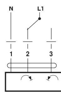
GR230G(..)-7
