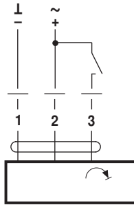
GR(C)24G(..)-5 GR24G(..)-7
