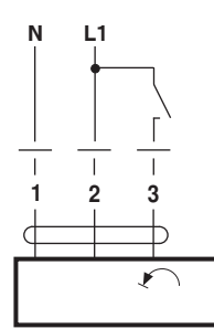
DR(C)230G(..)-5 DR(C)230G(..)-7
